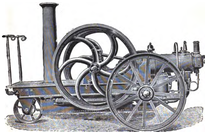
3. Керосиновый локомобиль Креслей 7 силъ.
